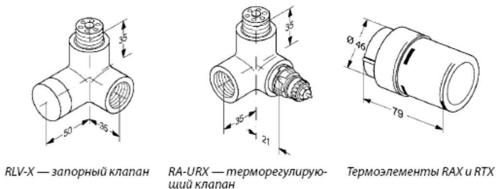
Рис. 3. Габаритные и присоединительные размеры
