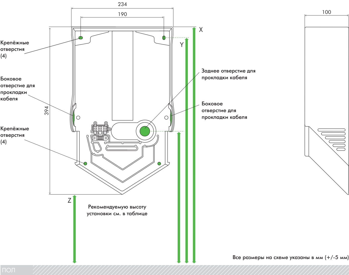
ВИД СЗАДИ
